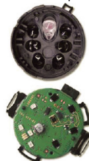
Type H2 (pluie/luminosité/ solaire) avec dispositif électronique
