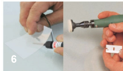
6 Nach dem Finish-Harz Auftrag wird überschüssiges Harz abgeschabt und die Reparaturstelle aufpoliert
