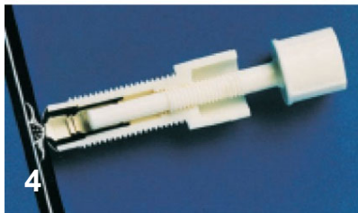
4 Das Füllharz wird unter Druck in die Einschlagstelle eingepresst, die Luft unter Vakuum entfernt
